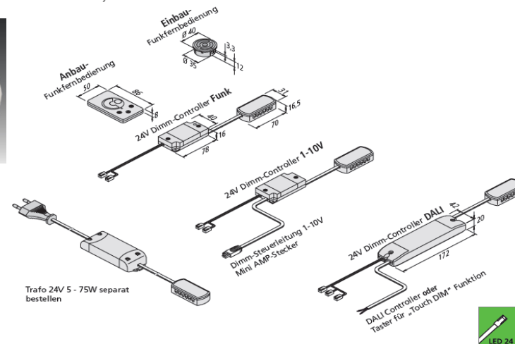
Dali Controller
