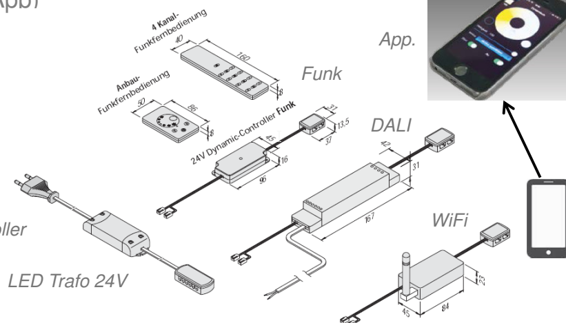
Einfache Baukastensystem: Trafo 24 V + Controller + Leuchte
